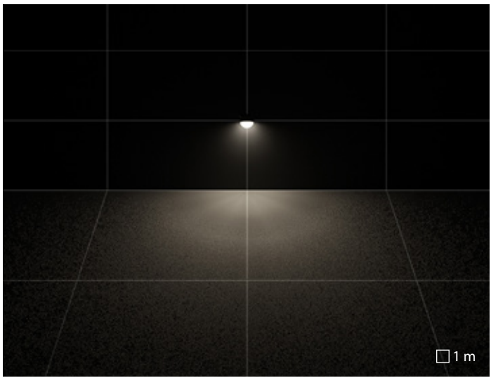
A/EW asymmetrische extra verspreidende
