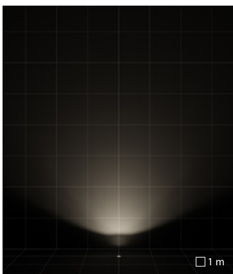
A5/M asymmetrische gemiddelde optiek
