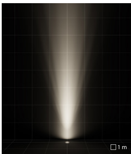
C/I cirkelvormige intensieve optiek
