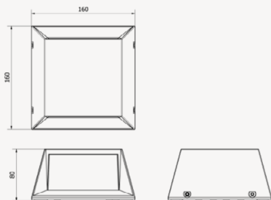
Afschermkap SYMM (afmetingen in mm)
