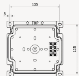
Montageplaat SYMM (afmetingen in mm)
