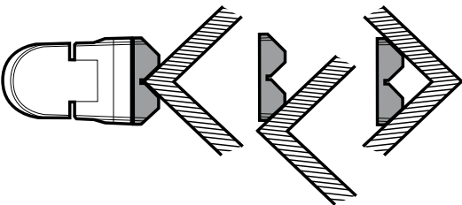
BINNEN- EN BUITENHOEKMONTAGE
