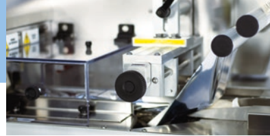
verstellbare Formschulter
