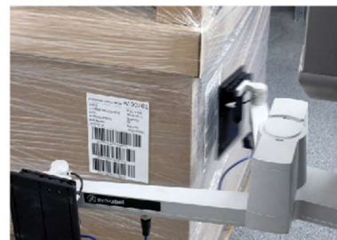
rotierender 360 ° FlexWipe Applikator
