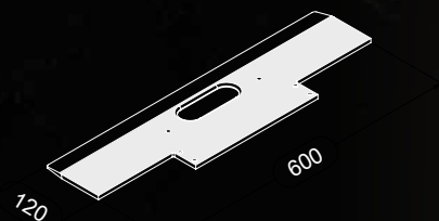
Schaufel 600 x 120 mm
