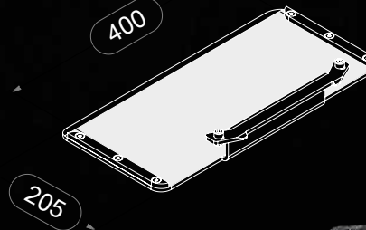
Einhängeschaufel für Getränkekisten 400 x 205 mm
