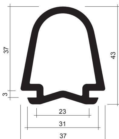
TT 1 (voir aussi TT 2) pour portes Delaval
