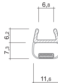
Set Nr. 16 90° DD0118SET 2010 mm
