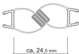
Set Nr. 25 180° DD0162SET 2010 mm
