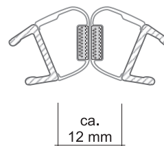
Set Nr. 18 135° DD0122SET 2010 mm
