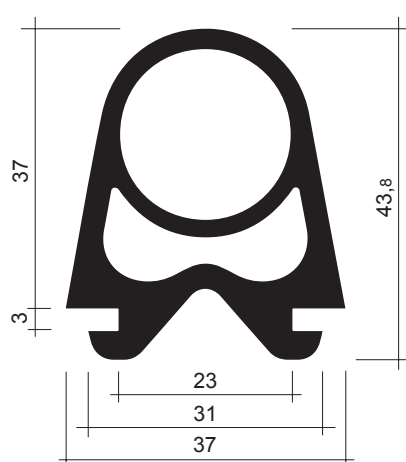
TT 2 (voir aussi TT 1)
