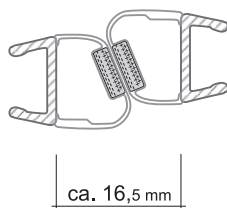
Set Nr. 19 180° DD0123SET 2010 mm
