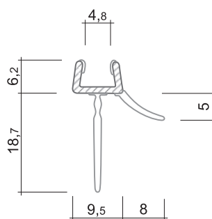
Set Nr. 26 180° DD0163SET 2010 mm
