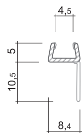
Set Nr. 24 90° DD0161SET 2010 mm
