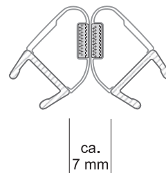
Set Nr. 16 90° DD0118SET 2010 mm
