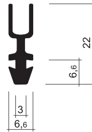
DD0142TR 1400 mm Produit n'est plus disponible
