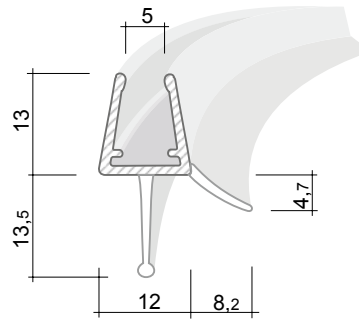
DD22 R 500 mm | DD23 R 550 mm
