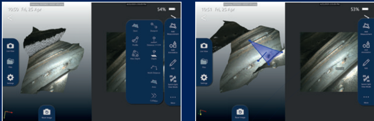
Messansicht mit 2D/3D Darstellung zur intuitiven Vermessung komplexer Bauteile
