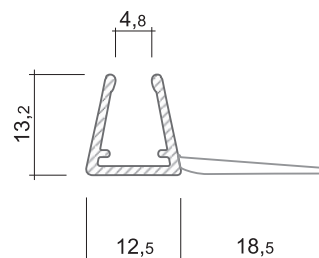
Set Nr. 13 180° DD0095SET 2010 mm
