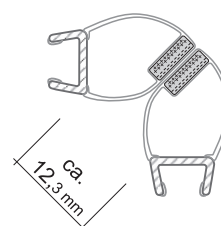
Set Nr. 24 90° DD0161SET 2010 mm
