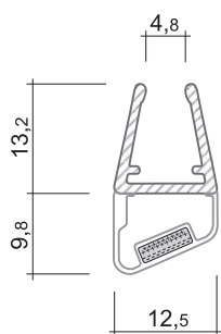
DD0092TR 2010 mm NS DD0093TR 2010 mm SN
