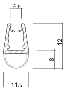
Set Nr. 27 180° DD0171SET 2500 mm
