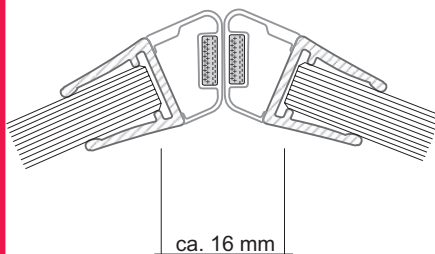
Set Nr. 12 135° DD0094SET 2010 mm
