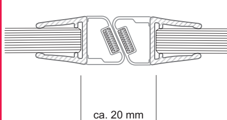
Set Nr. 13 180° DD0095SET 2010 mm
