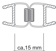
Set Nr. 15 180° DD0115SET 2010 mm
