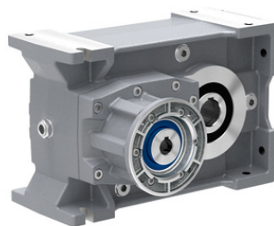
REDUCTORES EJES PARALELOS FUNDICIÓN
