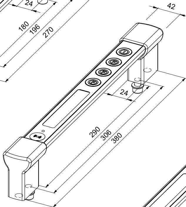
Funktionsgriff Grösse 2
