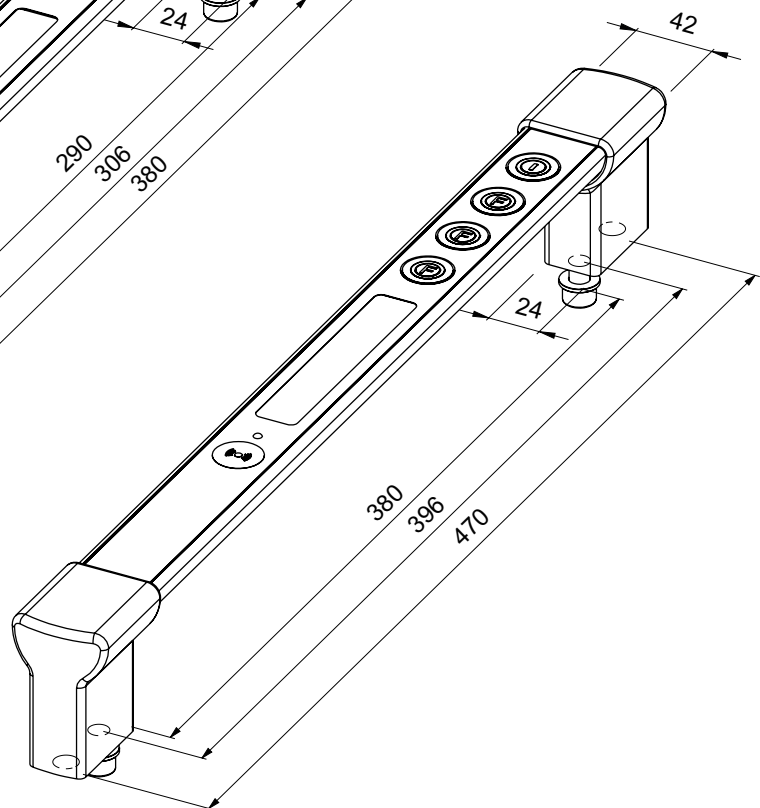
Funktionsgriff Grösse 3
