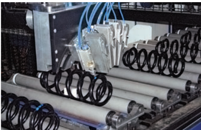
Kennzeichnung von Stahlfedern zur Typenklassifizierung
