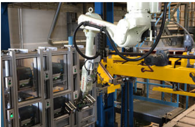
Flexibles Roboter Etikettiersystem
