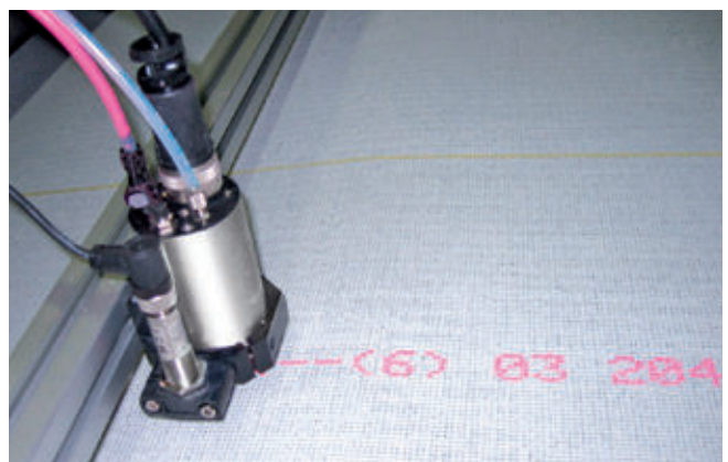
Kennzeichnung von Bahnenware
