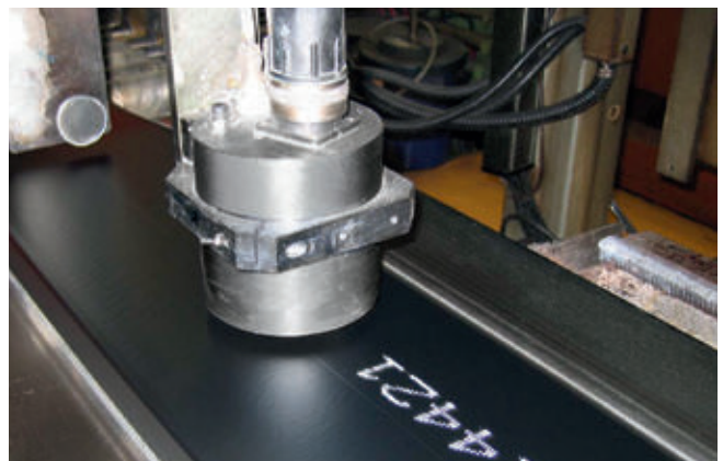
Laufstreifenkennzeichnung von Rohgummi
