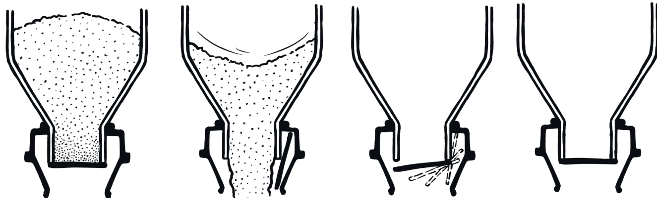
Bild 3: Schematische Darstellung der Klappenverschlussmechanik bei einer Vollentleerung
