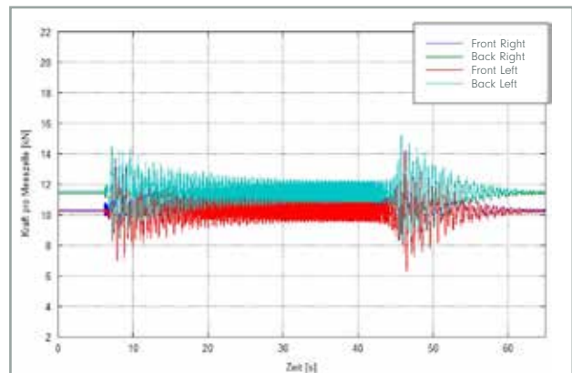
Abb 2 STEINHAUS Airsprings
