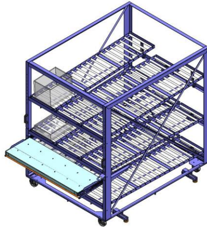
Kommissionierwagen mit einem Rollensystem
