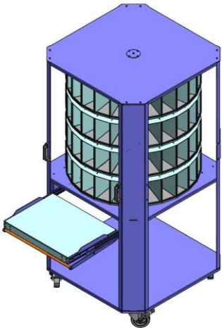
Kommissionierwagen mit Drehsäule
