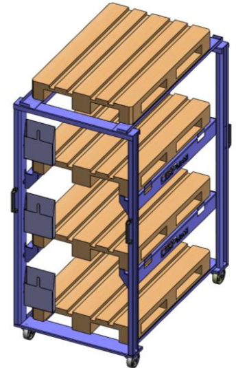
Kommissionierwagen mit Palettenaufnahme
