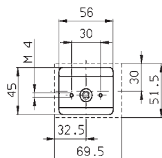
Schalterstirnseite Front view
