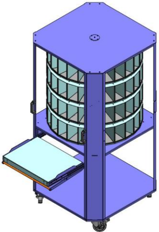
Kommissionierwagen mit Drehsäule
