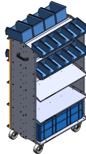
Kommissionierwagen mit Schüttenaufnahme
