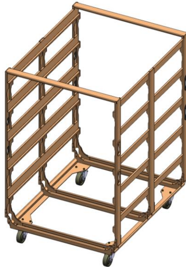
Mobiles Stapelregal
