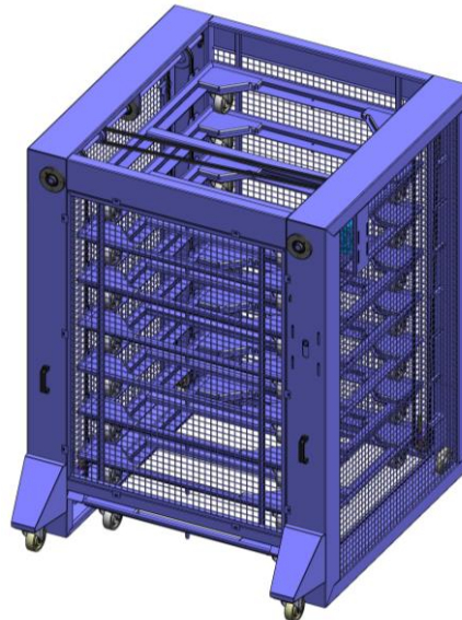
Mobile halbautomatische Ausführung
