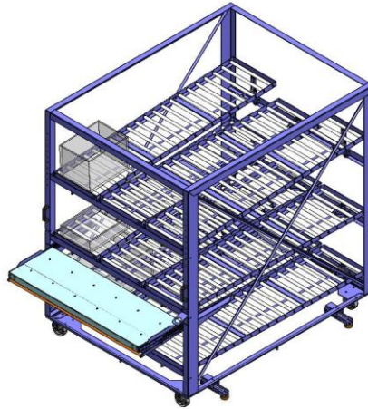
Kommissionierwagen mit einem Rollensystem
