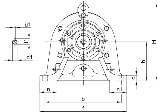
Horizontale Einbaulage
