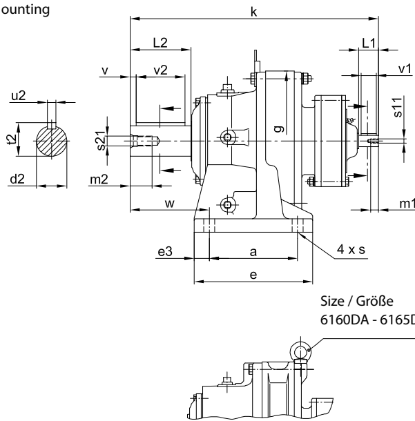
Horizontale Einbaulage
