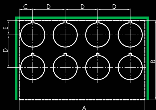
Basismodul
