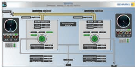
Prozessbild zu zwei BHKWs
