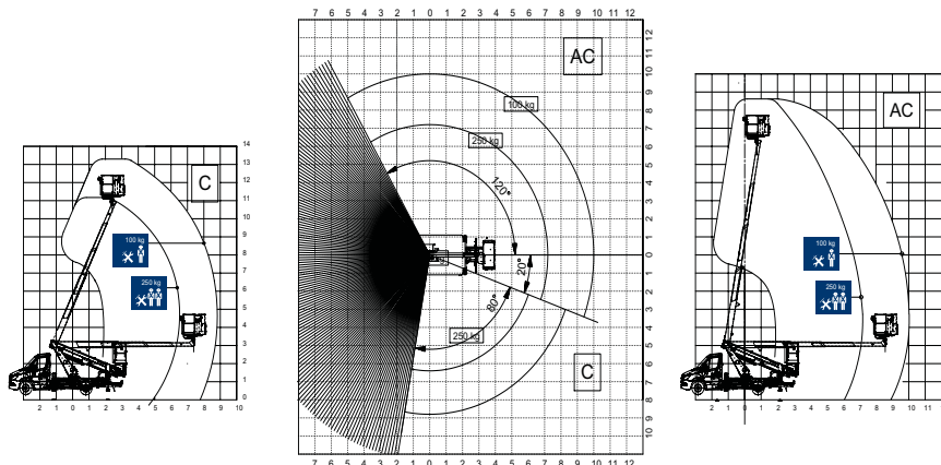
Stelpoten aan een zijde open en een zijde gesloten
