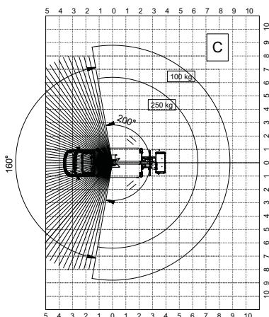
Stelpoten gesloten
