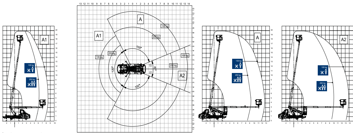
Stelpoten gesloten
