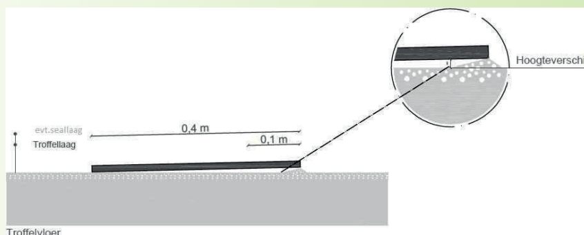
Afb. 5.3: Voorbeeld spaanslag
