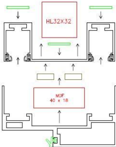
AANSLUITING DEURKADER-PLAFOND GROTE SCHADUWVOEG
