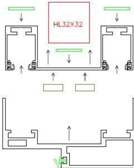
AANSLUITING DEURKADER-PLAFOND KLEINE SCHADUWVOEG
