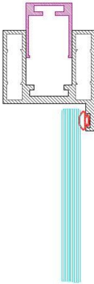
HORIZONTALE DOORSNEDE DETAIL ⑦ SCHAAL 1/1
