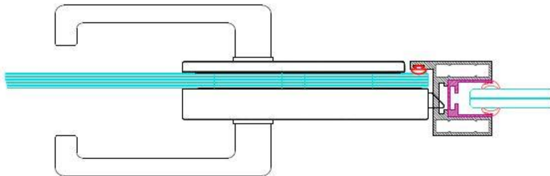
HORIZONTALE DOORSNEDE DETAIL ① SCHAAL 1/2
