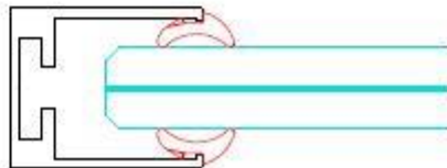
HORIZONTALE DOORSNEDE DETAIL (A) SCHAAL 1/1
