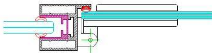
HORIZONTALE DOORSNEDE DETAIL ② SCHAAL 1/2
