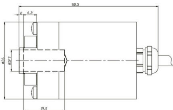
36W Axial
