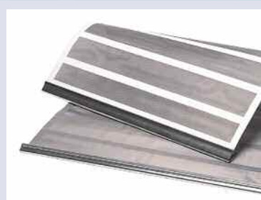
Mehrlagiger Siebboden, verstärkt mit PUR-Folie
