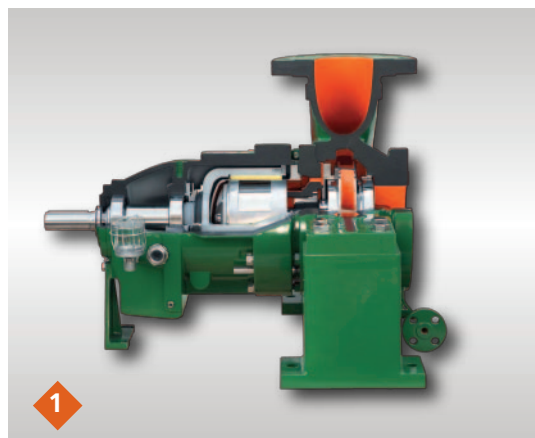
Centrifugaalpompe type PRM volgens API 685 Met magneetkoppeling.
