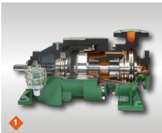
Centrifugaalpompe type NMR / NML / NMB volgens EN- en ISO-normen Met magneetkoppeling.
