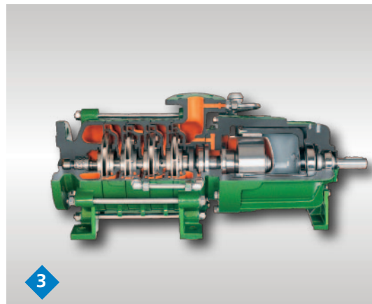
Meertraps centrifugaalpomp type HZ / HZM Met mechanische asafdichting of magneetkoppeling. Ook leverbaar in zelfaanzuigende uitvoering.
