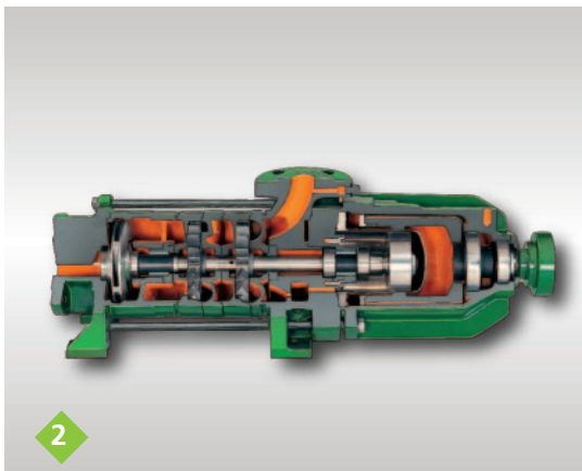
Zijkanaalpomp type SC / SCM Turbinepomp type YPM Met mechanische asafdichting of magneetkoppeling.
