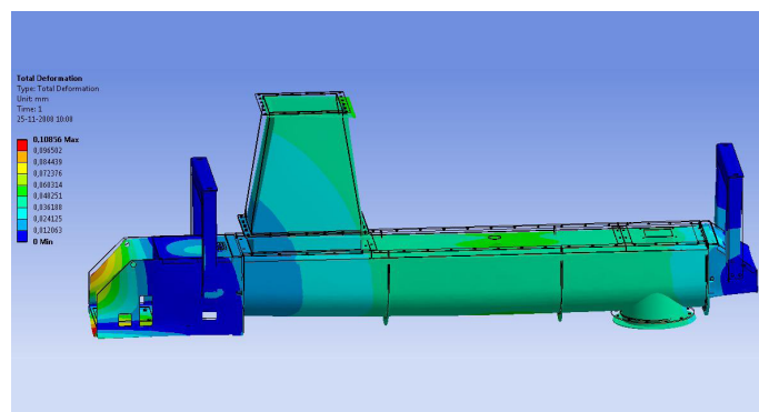
Sterkteberekening trogtransporteur
