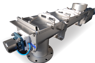
Trogtransporteur met scharnierende deksels welke 100% stofdicht zijn inwendig heerst een overdruk van 200 mbar
