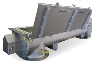
Trogtransporteurs voor de voedingsmiddelenindustrie snelreinigbaar door scharnierende deksels
