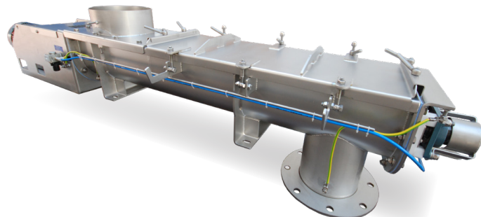
Trogtransporteur voorzien van sperlucht aansluiting op de as afdichtingen
