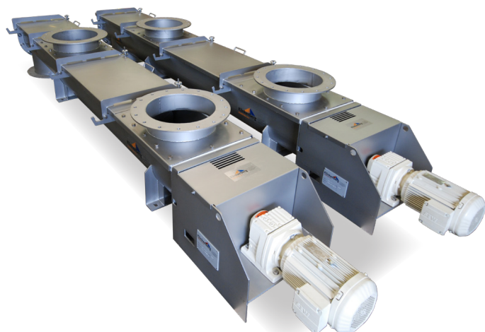
Trogtransporteur uitgevoerd met twininlaat
