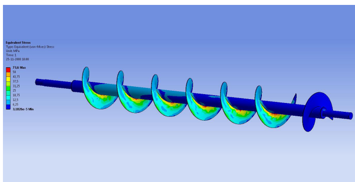
Sterkteberekening schroefas
