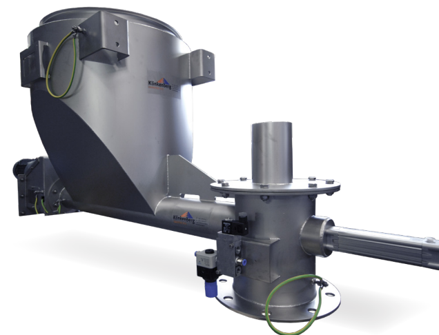
Pneumatische kopklepschroef met 1000 liter hopper Zone 20 inwendig uitwendig Zone 22
