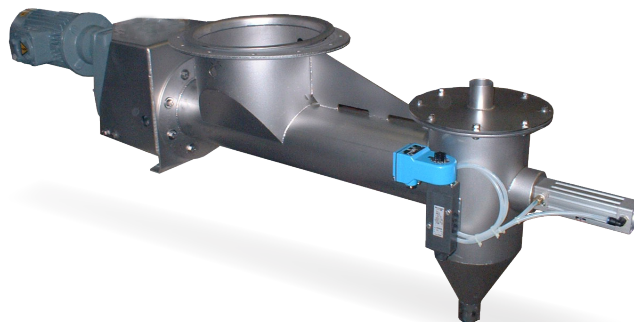
Kopklep/doseerschroefje voor het doseren van granulaat, direct in pneumatisch transport.
