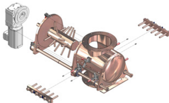
Enkele pennenbreker welke snelreinigbaar is uitgevoerd. Goed inzetbaar bij bedrijven waar veel productwissels aan de orde zijn.
