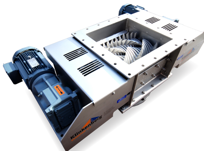
Twee assen aangedreven messenbreker voor het breken van zeer harde agglomeraten. Per as is een aandrijving voorzien.
