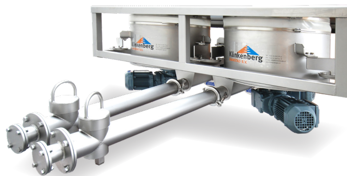
Gewogen doseersysteem met dubbele agitator en twee doseerschroeven uitgevoerd met opleg/snijtafel voor het snijden van 25kg zakken
