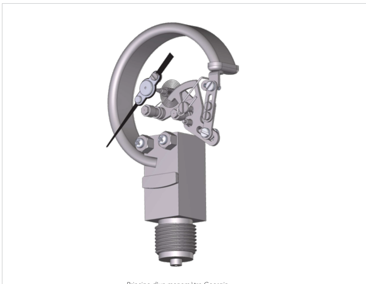
Principe d'un manomètre Georgin
