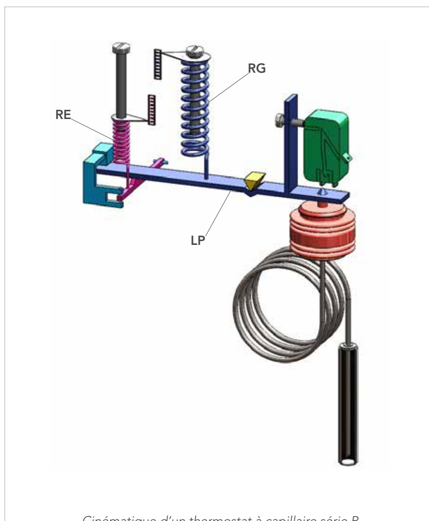
Cinématique d'un thermostat à capillaire série P
