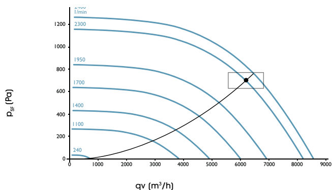
Luchtstroom p_{sf}
