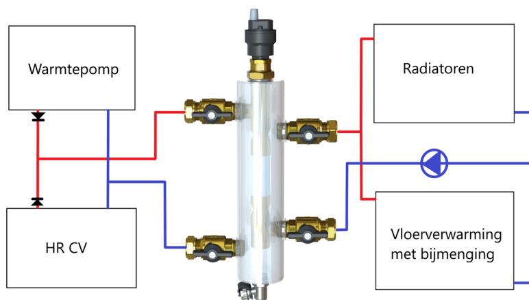
Schematische weergave Open Verdeler
