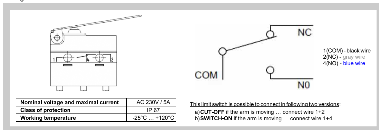
Fig. 6 Limit switch G905-300E03W1
