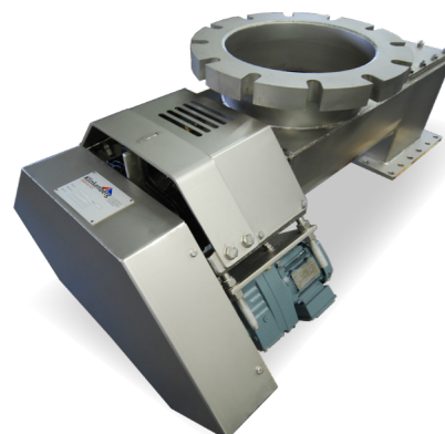
Massastroom doseren van houtpallets uit torrefactie proces Volledig ontwikkeld om een massastroomproces te garanderen
