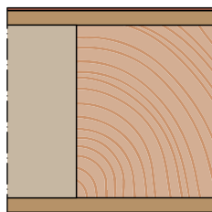
Houten kader (vanaf deurdikte 60)
