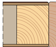
Zichtbare houten kantlat (vanaf deurdikte 50)
