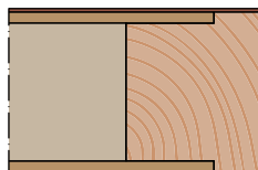
Couvre-chant sur collée en bois (jusqu'à l'épaisseur de porte 50)
