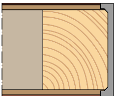
Couvre-chant visible moulé - PU Ne peut être moulée qu'en combinaison d'un HPL sans relief (à partir de l'épaisseur de porte 50)
