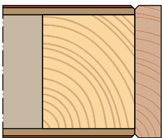
Couvre-chant visible en bois (à partir de l'épaisseur de porte 50)
