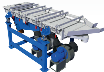
VRU HYBRID Vibrovaglio rettangolare VRU HYBRID Vibrating cooler VRU HYBRID
