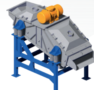
VRR Vibrovaglio rettangolare VRR Rectangular Screener VRR
