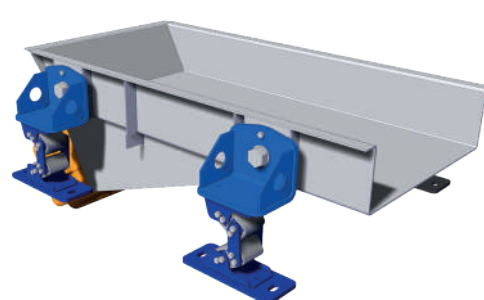
AV-M Alimentatore Elettromagnetico AV-M. Electromagnetic Feeder AV-M
