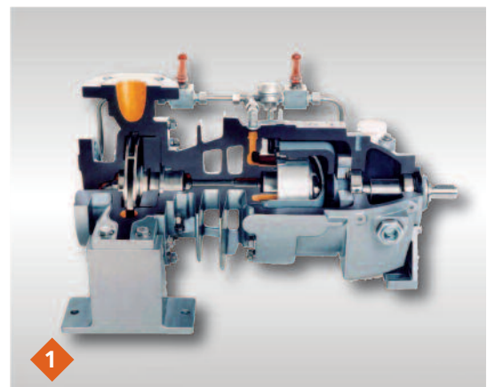
Centrifugaalpompe type NMWR / PRMW voor thermische olie Met magneetkoppeling voor temperaturen tot 450°C.
