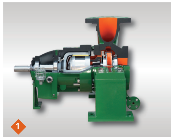
Centrifugaalpompe type PRM volgens API 685 Met magneetkoppeling.
