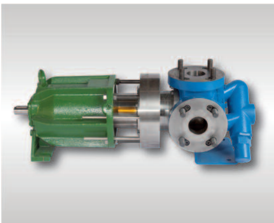
Tandradpompe type GML / GMB Met magneetkoppeling.
