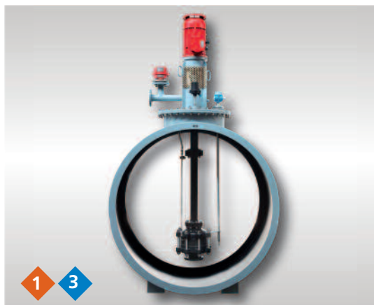
Verticale één- of meertraps staartpompe type NCT / HZV / NMT Met mechanische asafdichting of magneetkoppeling. Geschikt voor ATEX Zone 0.
