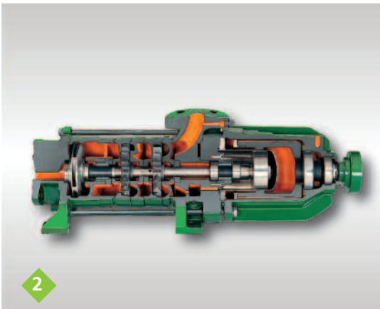
Zijdekanaalpompe type SC / SCM Met mechanische asafdichting of magneetkoppeling.
