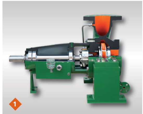
Centrifugaalpompe type NCR volgens API 610 Met mechanische asafdichting.
