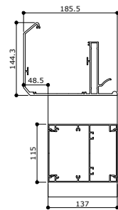
Gouttière classique
