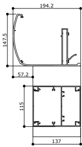
Gouttière arrondie
