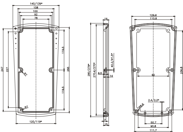
Lid frame
