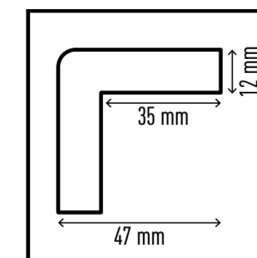
Hoekbeschermingsprofiel C35 #1112-130 - magnetisch
