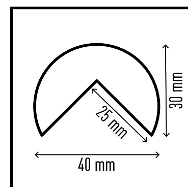
Hoekbeschermingsprofiel C25R #1110-130 - magnetisch
