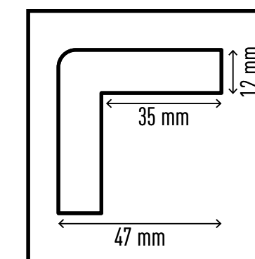
Profilé de protection d'angle C35 #1112-130 - magnétique
