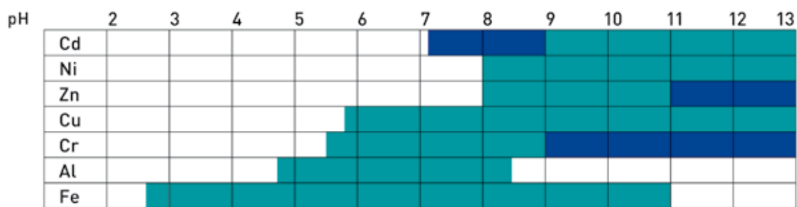
Standaard pH waarden voor zware metalen precipitatie Uitgebreide pH waarden met Neutralac®
