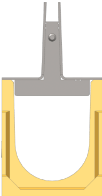
■ Fineline opzetelement gecombineerd met G100 lijngoot
