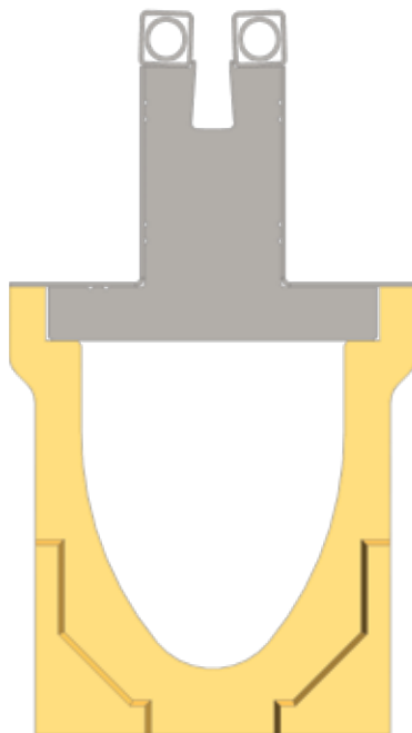
■ Squareline opzetelement gecombineerd met BasicDrain lijngoot
